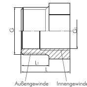
Außengewinde Innengewinde
