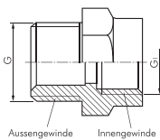
Aussengewinde Innengewinde
